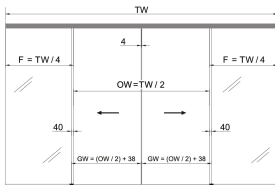
TW : Total width OW : Opening width GW : Glass panel width F : Fixed panel width
