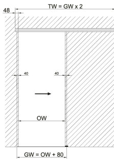
TW : Total width OW : Opening width GW : Glass panel width
