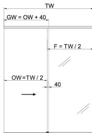
TW : Total width OW : Opening width GW : Glass panel width F : Fixed panel width
